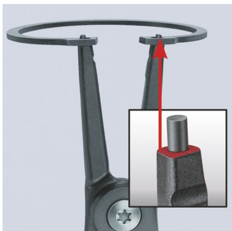
KNIPEX precisionslåsringsång: torsionsfri, lätt och snabb montering av ringen
