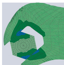
Tångnyckel: ytpressning utan spel, inga skador på kanter
